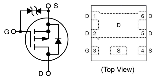
P-CHANNEL MOSFET
