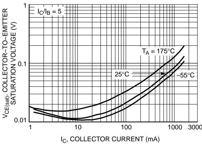
Figure 6. VCE(sat) - IC
