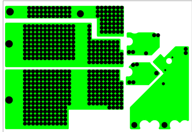
Layer 2, Internal
