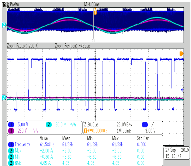
Figure 27. Vin = 220 Vac, Vo = 400 V, Iin = 20 A
