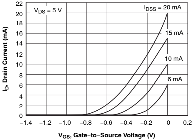
Figure 3. I_D - V_{GS}
