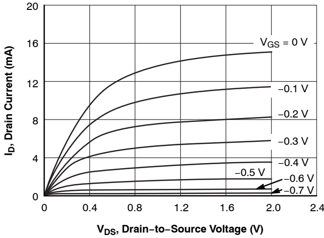
Figure 1. I_D - V_{DS}
